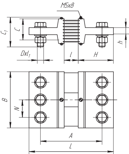
Рис. 13 75ШИС (5000 А, 6000 А)
