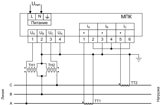
Трехфазное трехпроводное двухэлементное подключение с использованием 2 ТТ и 2 ТН
